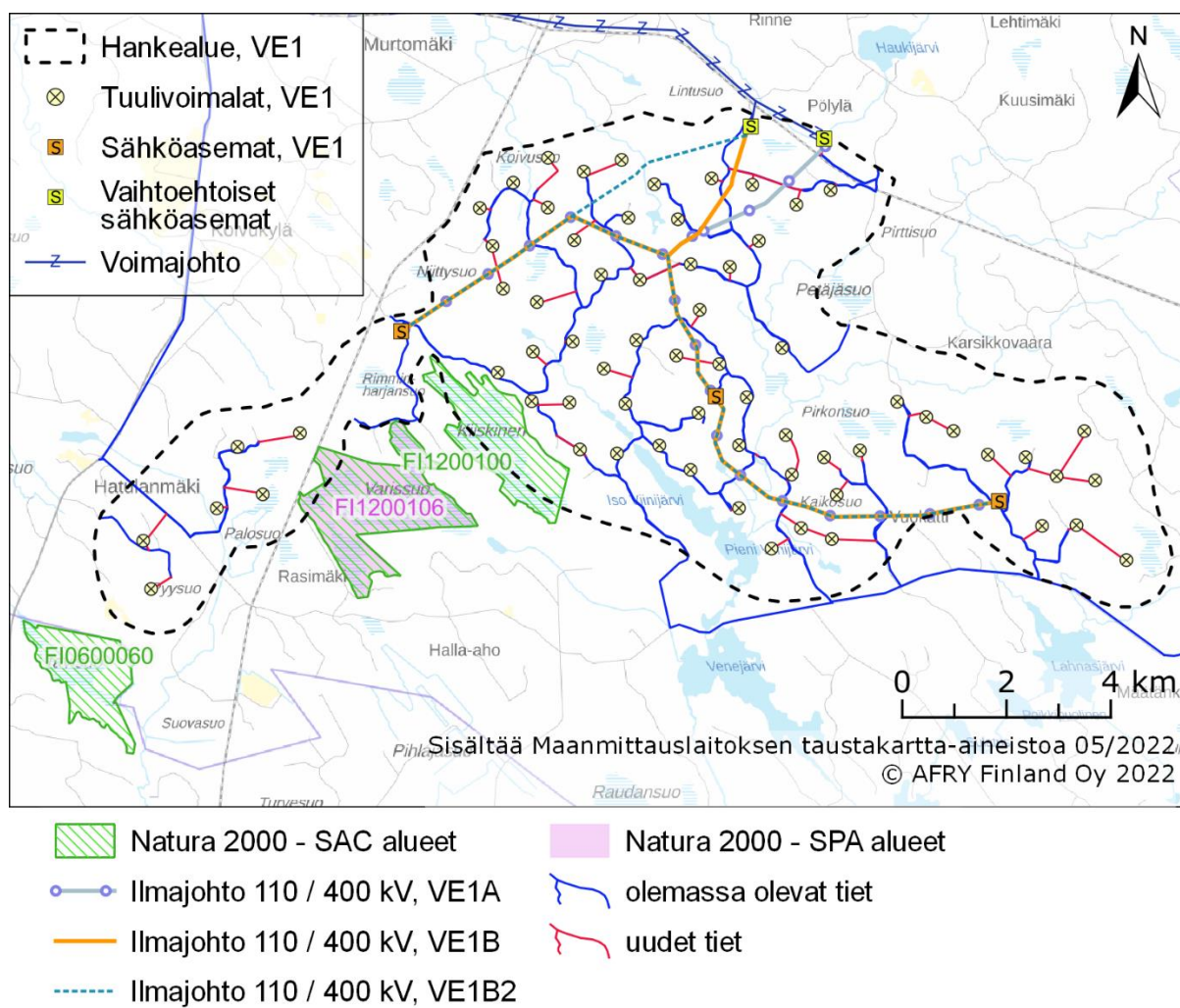
Kuva 2-1 VE1:n mukainen tuulipuiston sijoitussuunnitelma.
